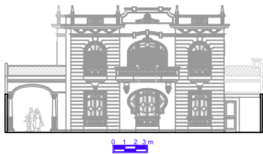
Elevation 01
