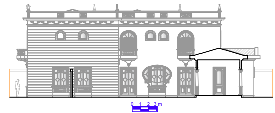
Elevation 04
